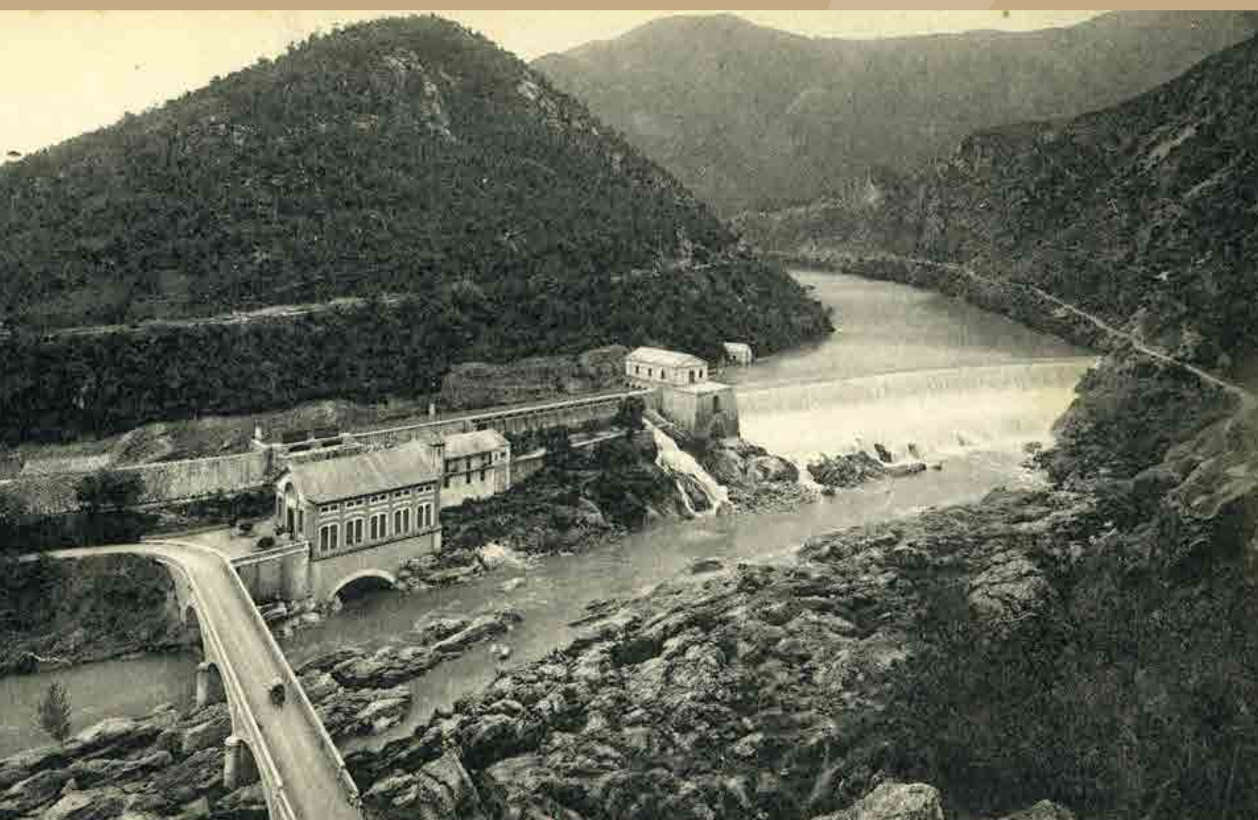
El massís de les Guillerries va ser un magnífic refugi per als carlins. En les imatges, el pas del Pasteral abans i després de la construcció de la presa, molt a prop de l'indret on va tenir lloc una de les batalles més decisives de la Segona Guerra Carlina (1846-1849).
